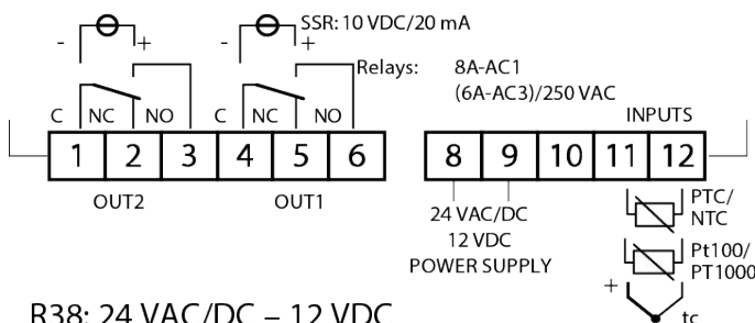
Fig. 5 PTC / NTC / PT1000 input wiring
