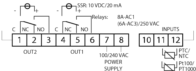
Fig. 4 PT100 input wiring
